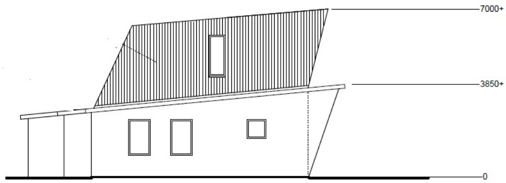
AANZICHT RECHTERZIJGEVEL (HEEMSKERKLAAN)
