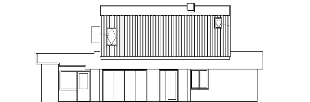
AANZICHT ENTREEGEVEL (VOORGEVEL VAN KINSBERGENLAAN)
